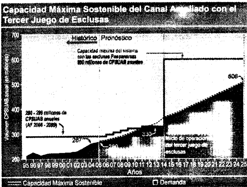
Figura 27 Con el tercer juego de esclusas el Canal ampliado podrá transitar más de 600 millones de toneladas CPSUAB anuales. Esto representa aproximadamente el doble de la capacidad máxima sostenible del Canal actual, suficiente para atender la demanda más allá del 2025.
