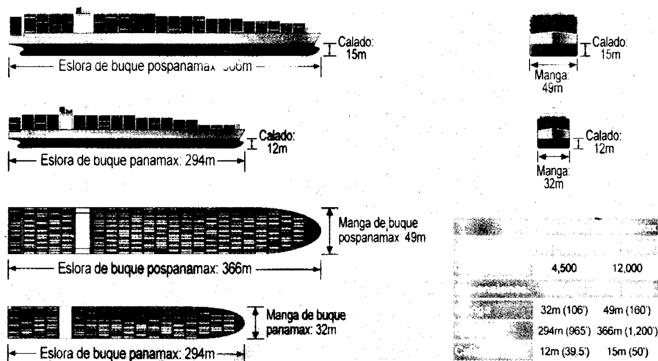
Figura 30 Comparación entre un buque portacontenedores Panamax con las dimensiones máximas para transitar el Canal y un buque de dimensiones pospanamax de 12,000 contenedores. El nuevo buque tendría hasta 2.5 veces la capacidad de carga del actual buque Panamax.
